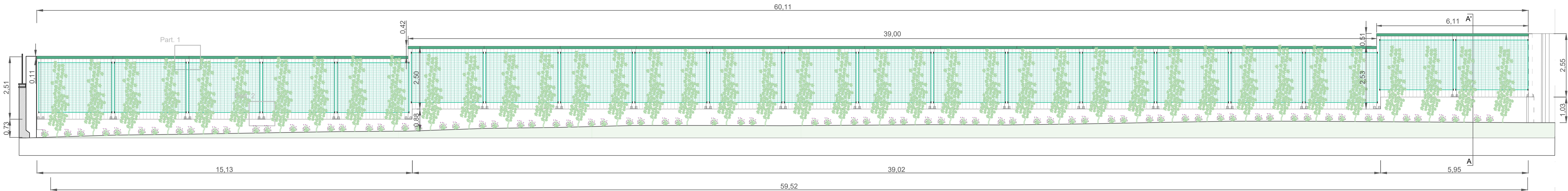
Prospetto- stato di progetto
