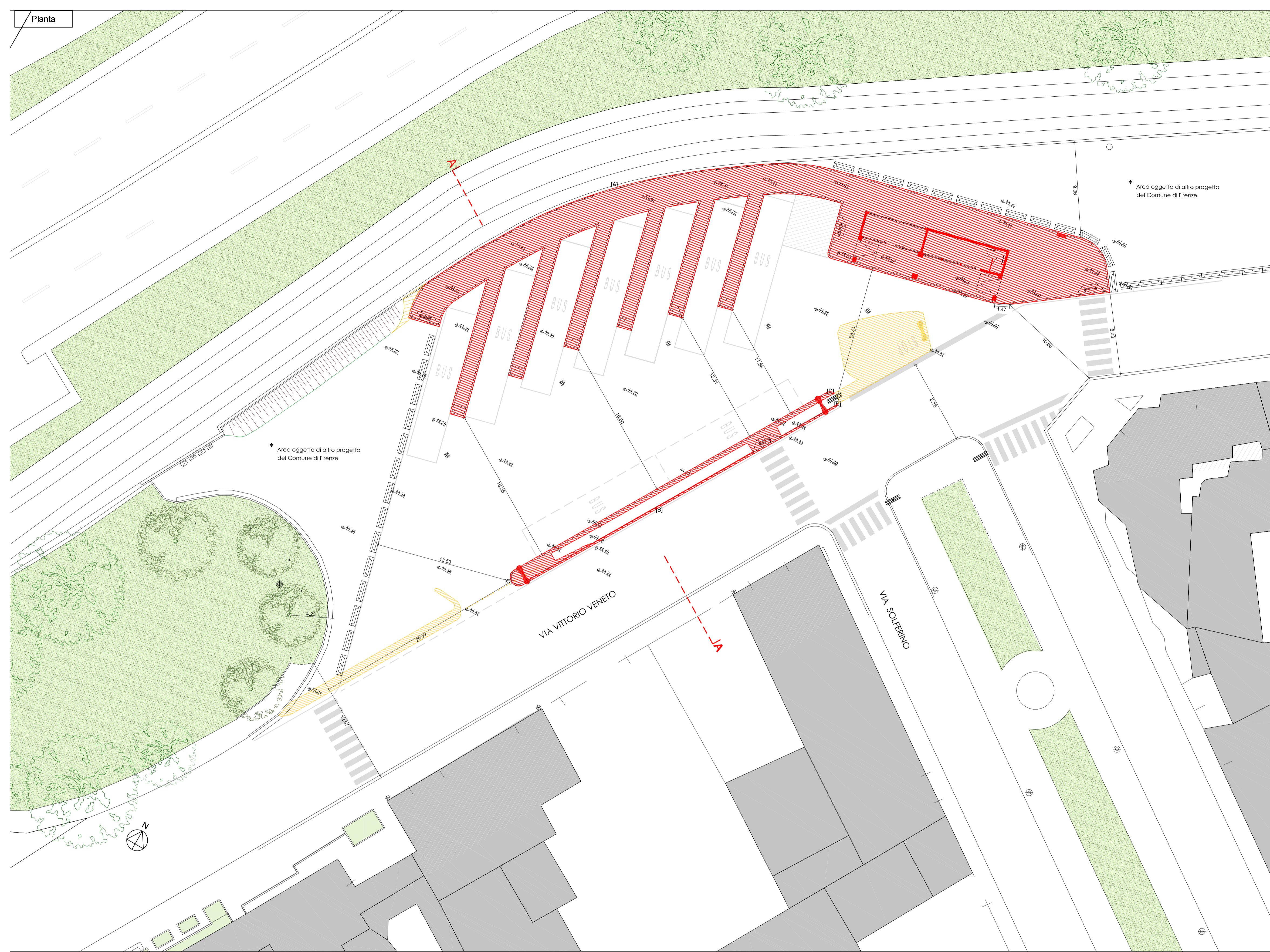
Sezione AA
