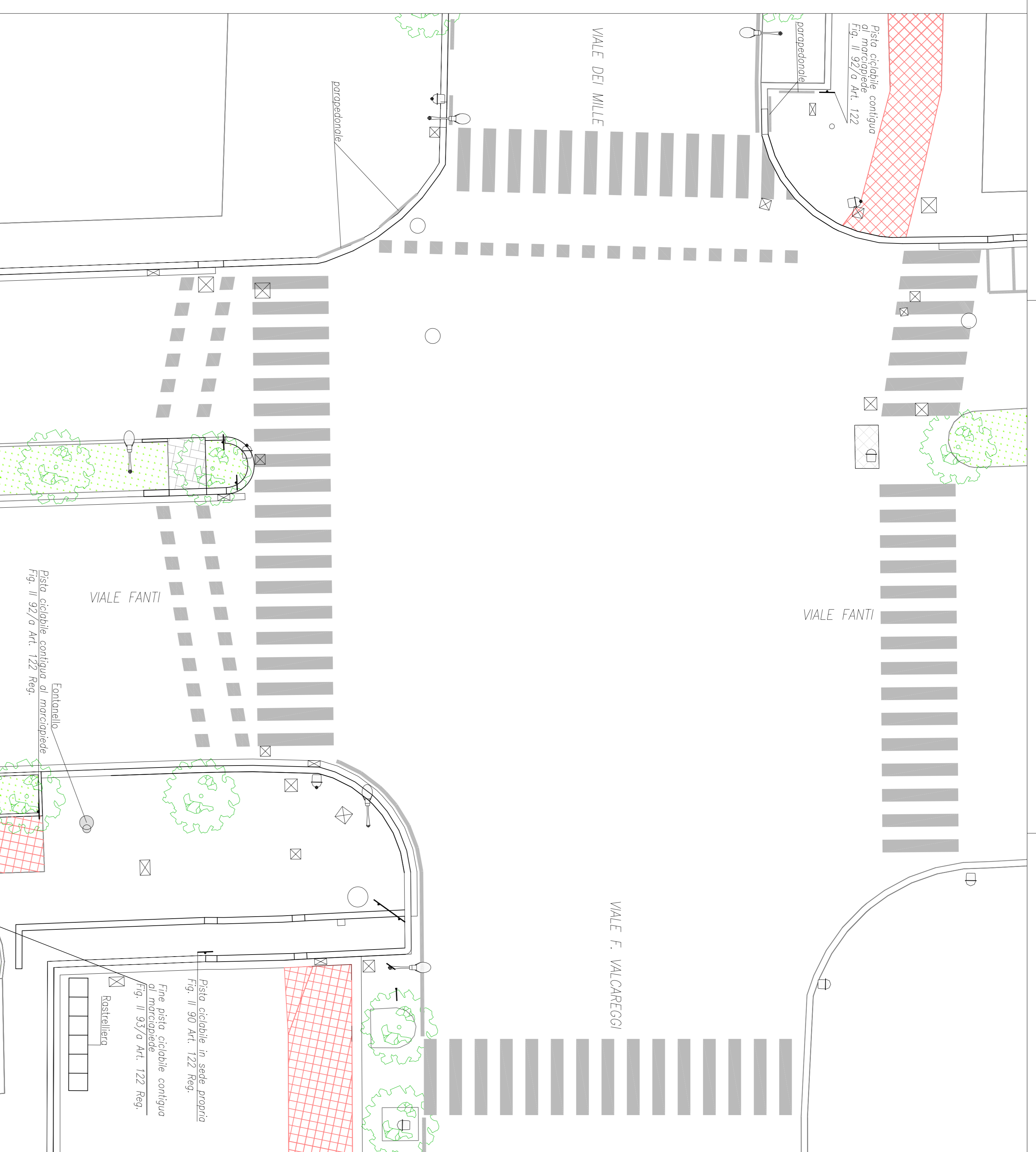
STATO DI FATTO SCALA 1:200
