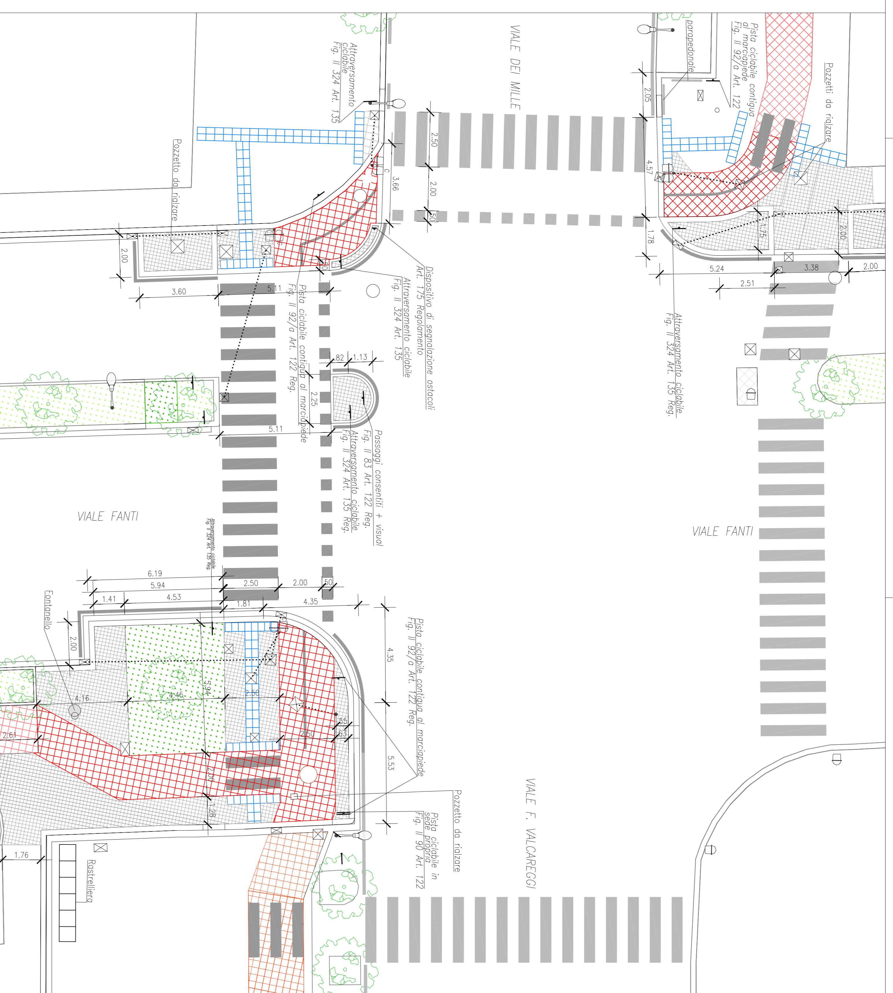
STATO DI PROGETTO SCALA 1:200
